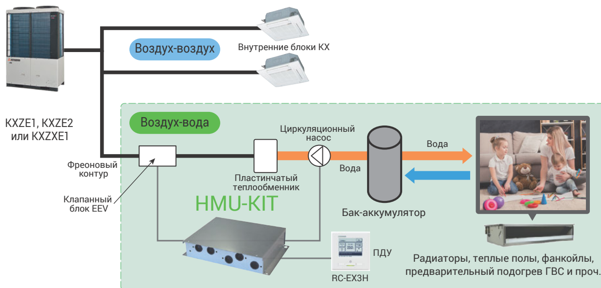
RC-EX3N контроллер для НМУ-КИТ
